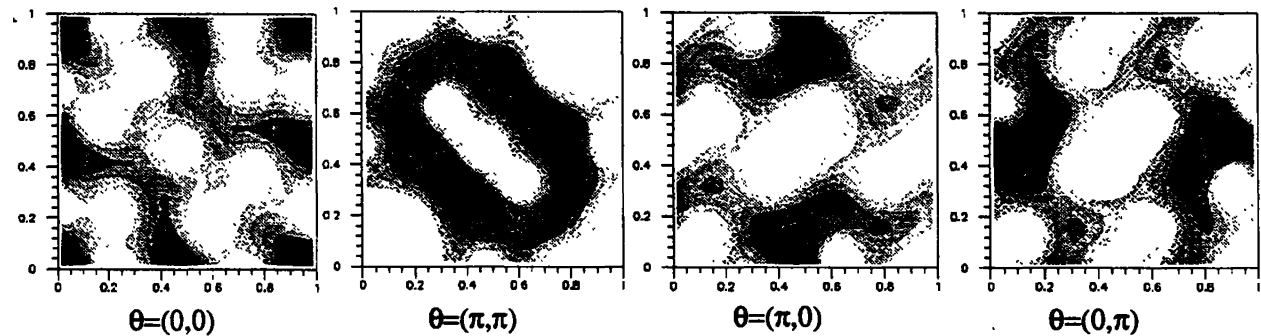
Figure 25: Distribution de Husimi de la bande \Psi_3 pour \gamma = 0.88 , ayant un indice de Chern C = 0 . La distribution fluctue néanmoins avec \bar{\theta} .
