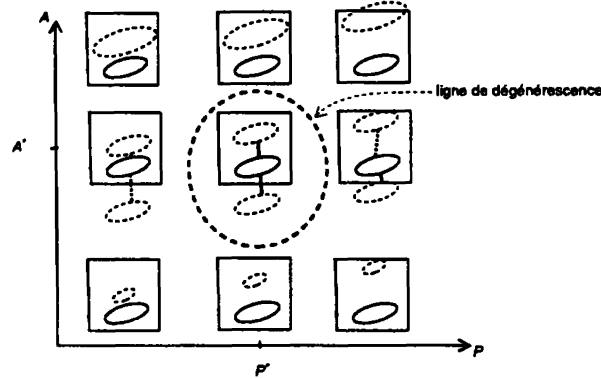
Figure 18: Diagramme montrant deux familles de trajectoires contractibles (au voisinage de E = \mathcal{H}(q,p) ), pour un Hamiltonien dépendant de deux paramètres (\mathcal{A}, \mathcal{P}) . L'indice de Chern est C = \pm 1 dans un voisinage de (\mathcal{A}^*, \mathcal{P}^*) limité par une ligne fermée de dégénérescence. Hors de laquelle C = 0 .
