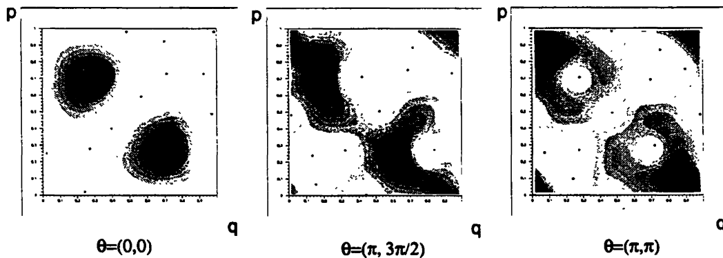
Figure 23: Distribution de Husimi de la bande \Psi_4 , \gamma = 0.66 . N = 11 d'indice de Chern C = 1 . (la bande \Psi_4 est indiquée par un cercle sur la figure (21)). On observe que la distribution fluctue entre le point fixe instable (q, p) = (0, 0) et la trajectoire périodique stable (q, p) = (0.7, 0.25) . Pour (\theta_1, \theta_2) = (\pi, 3\pi/2) la distribution est une superposition des deux autres distributions.
