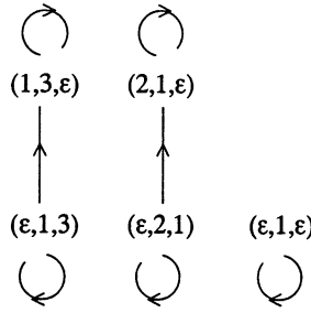
FIGURE 2. ordre \prec pour \sigma : 1 \mapsto 21, 2 \mapsto 13, 3 \mapsto 1
