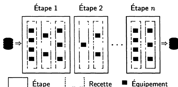
FIG 3. — Schématisation du processus de fabrication qui reçoit en entrée des lots de plaquettes vierges de silicium sur lesquelles sont intégrés les circuits au cours de cent à deux cents étapes durant un temps de cycle d'une dizaine de semaines.
