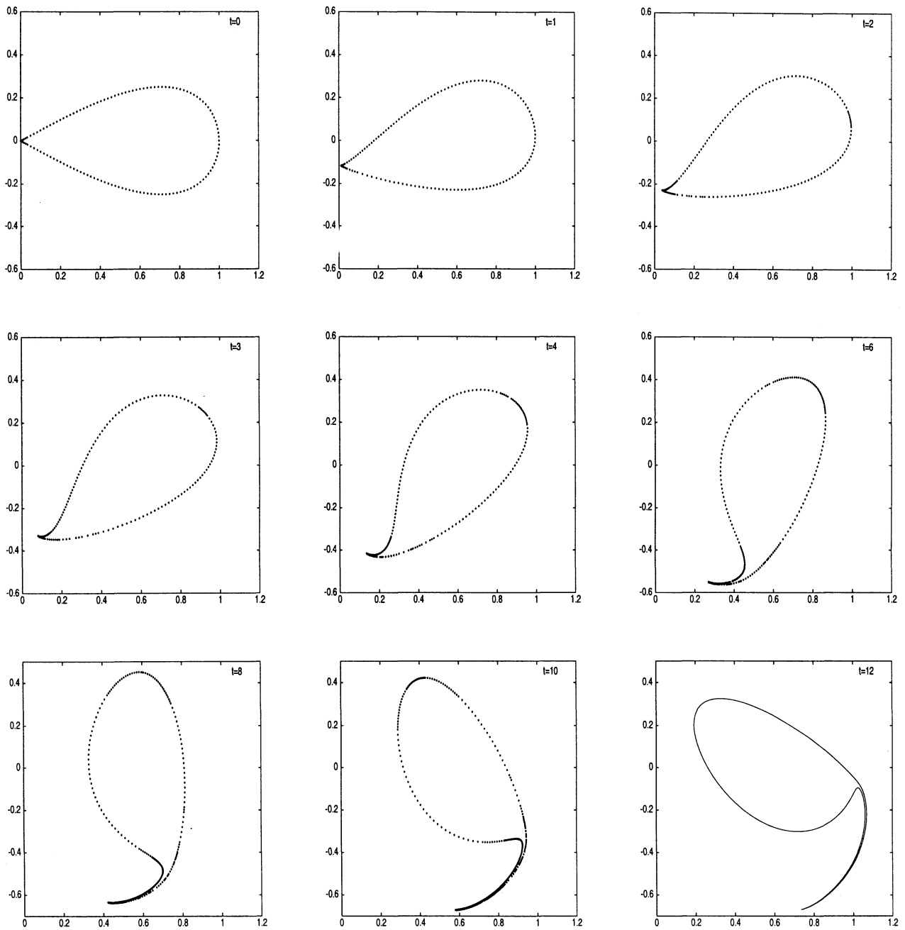
Fig. 1 : Évolution d'un angle aigu dans une poche de tourbillon. On a choisi \Delta t=0.04 et \epsilon=10^{-6} . Pour t=0, 1, 2, 3, 4, 6, 8 et 10 , la courbe a été représentée à l'aide des points effectivement utilisés pour calculer l'évolution. Pour t=12 , on a pris une grille fine de 32768 points.
