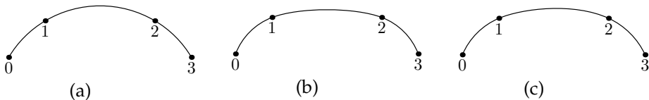
FIG. 10 – Résultats de draw z0..z1..tension \alpha and \beta ..z2..z3 pour différentes valeurs de \alpha et \beta : (a) \alpha = \beta = 1 ; (b) \alpha = \beta = 1.3 ; (c) \alpha = 1.5, \beta = 1
