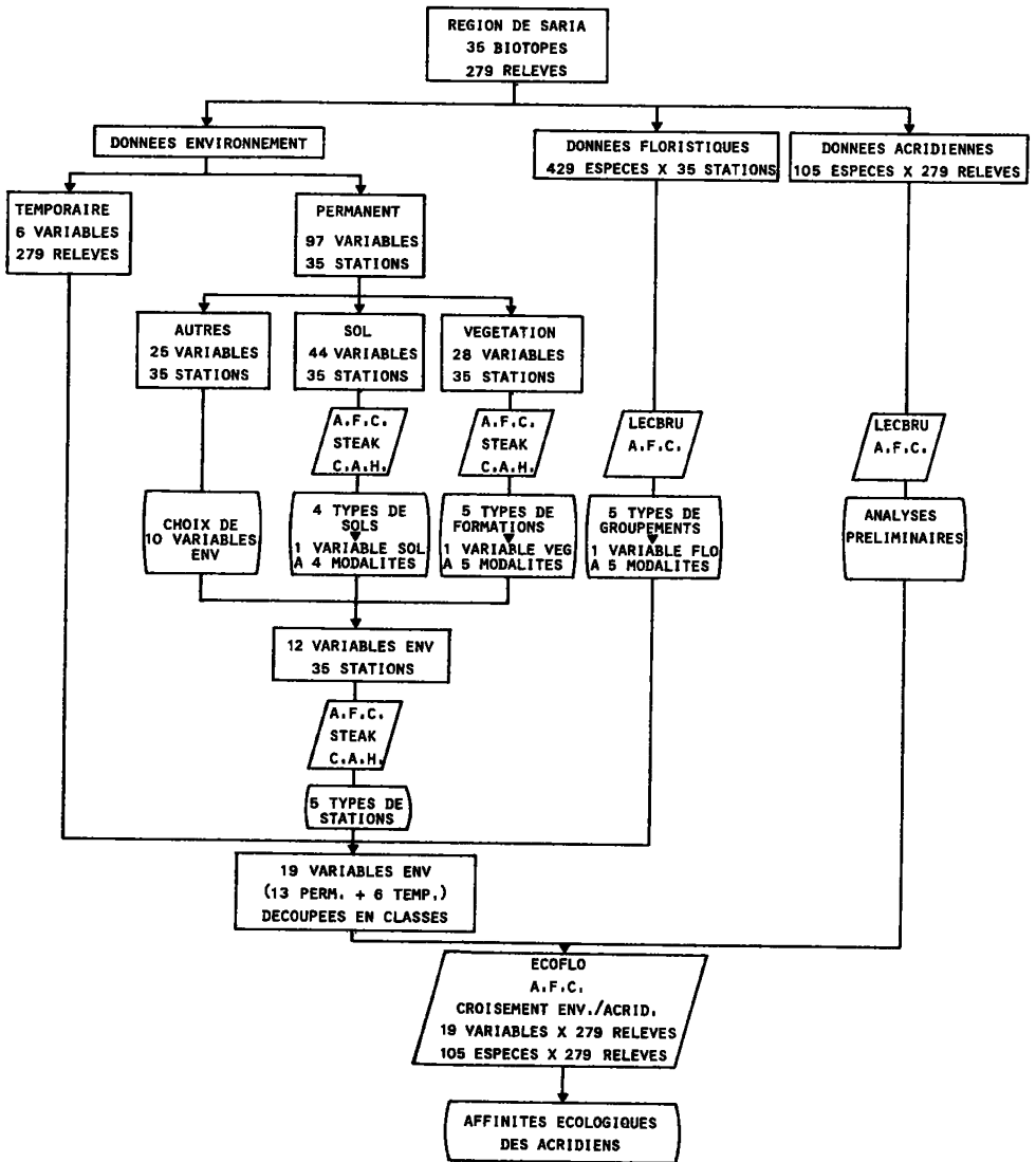
Figure 1 : Organigramme général du traitement des données A.F.C. : Programme d'analyse factorielle des correspondances C.A.H. : Programme de classification ascendante hiérarchique
