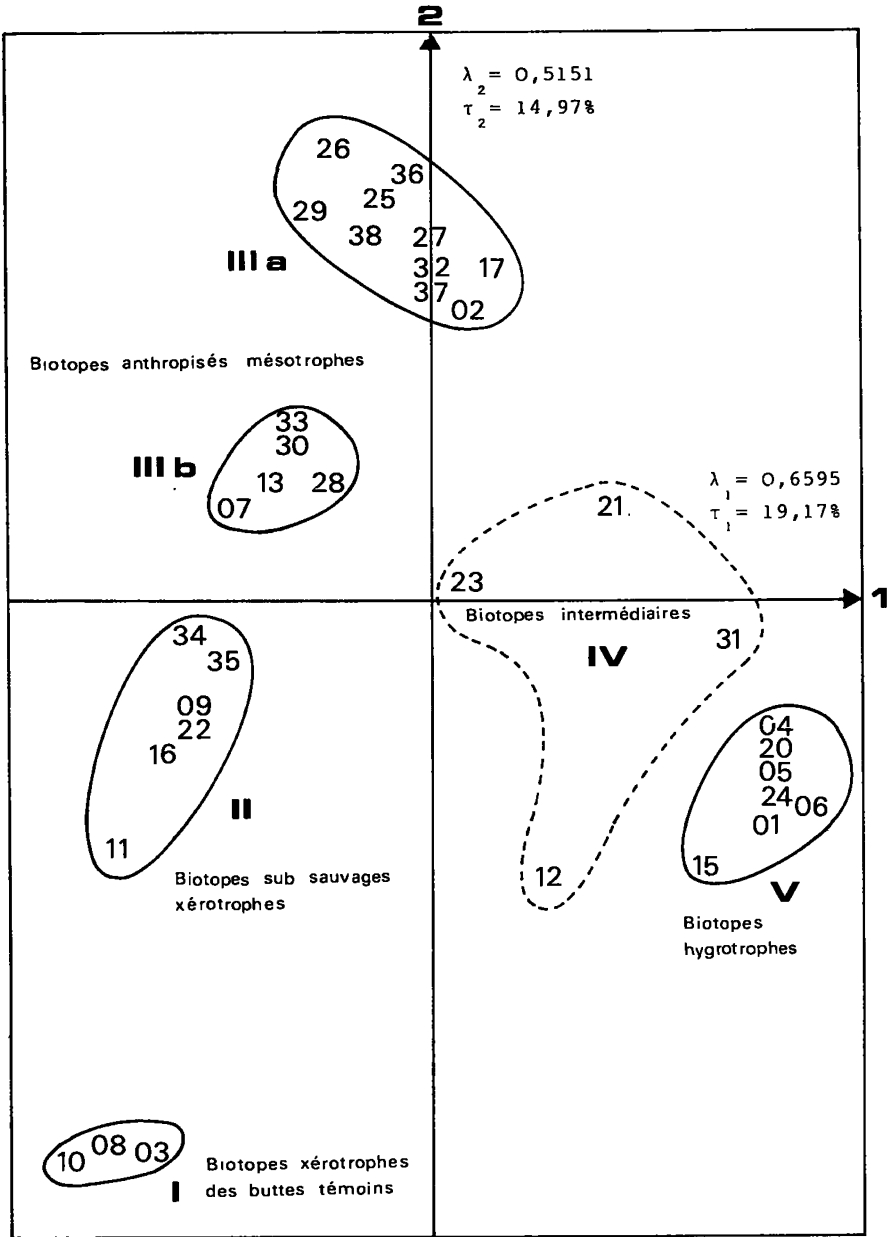
Figure 4 : Résultats de l'analyse des données sur l'environnement (12 variables (54 modalités) × 35 stations). Répartition des stations dans le plan des axes 1 et 2.
