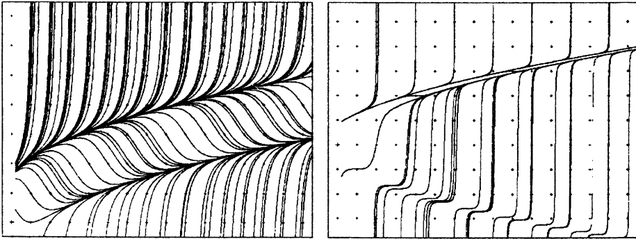
Figure 2: Partie gauche: équation Y' = (Y - \sqrt{X} - 1)(Y - \sqrt{X} + 1) . Il y a deux branches d'isocline 0, chacune d'elle correspond à une structure de type "fleuve singulier". Partie droite: équation Y' = (Y^2 - X)^2 . Il y a deux branches d'isocline 0, une d'entre elle ne correspond à aucun fleuve, l'autre à une paire attractif/répulsif.
