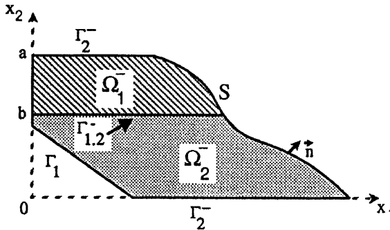
Fig. 2. - \Omega^- domain.
