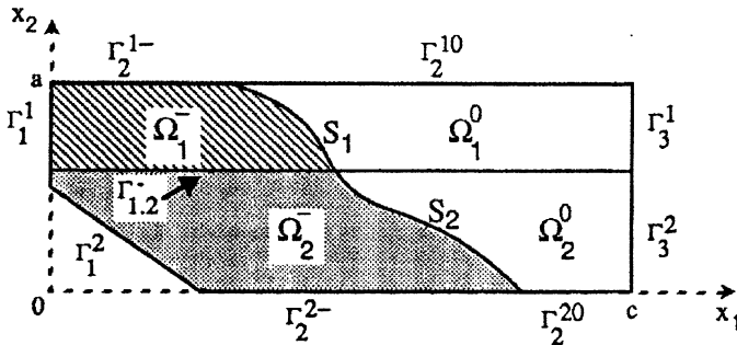
Fig. 3. - \Omega domain.
