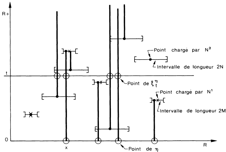
FIG. 1. — x : point chargé par N^1 ; • : point chargé par N^2 .
