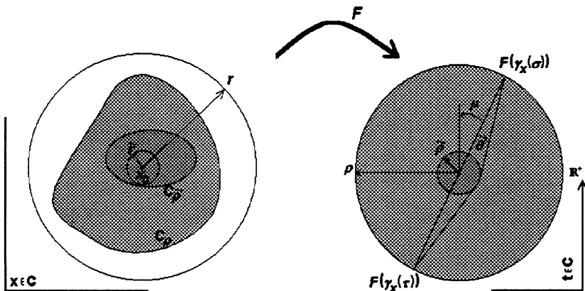
Fig. 2 Les régions de C_\rho et C_{\tilde{r}} comprises entre les disques de rayon r et \tilde{r} et leurs images par F .
