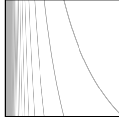
1/x-y \text{ entier } >0 \text{ (ou } x=0)
